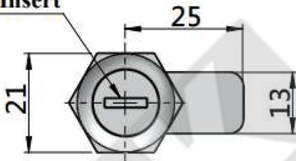
Slot Insert
